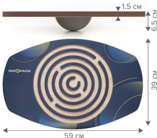
Рис. Устройство балансборда
