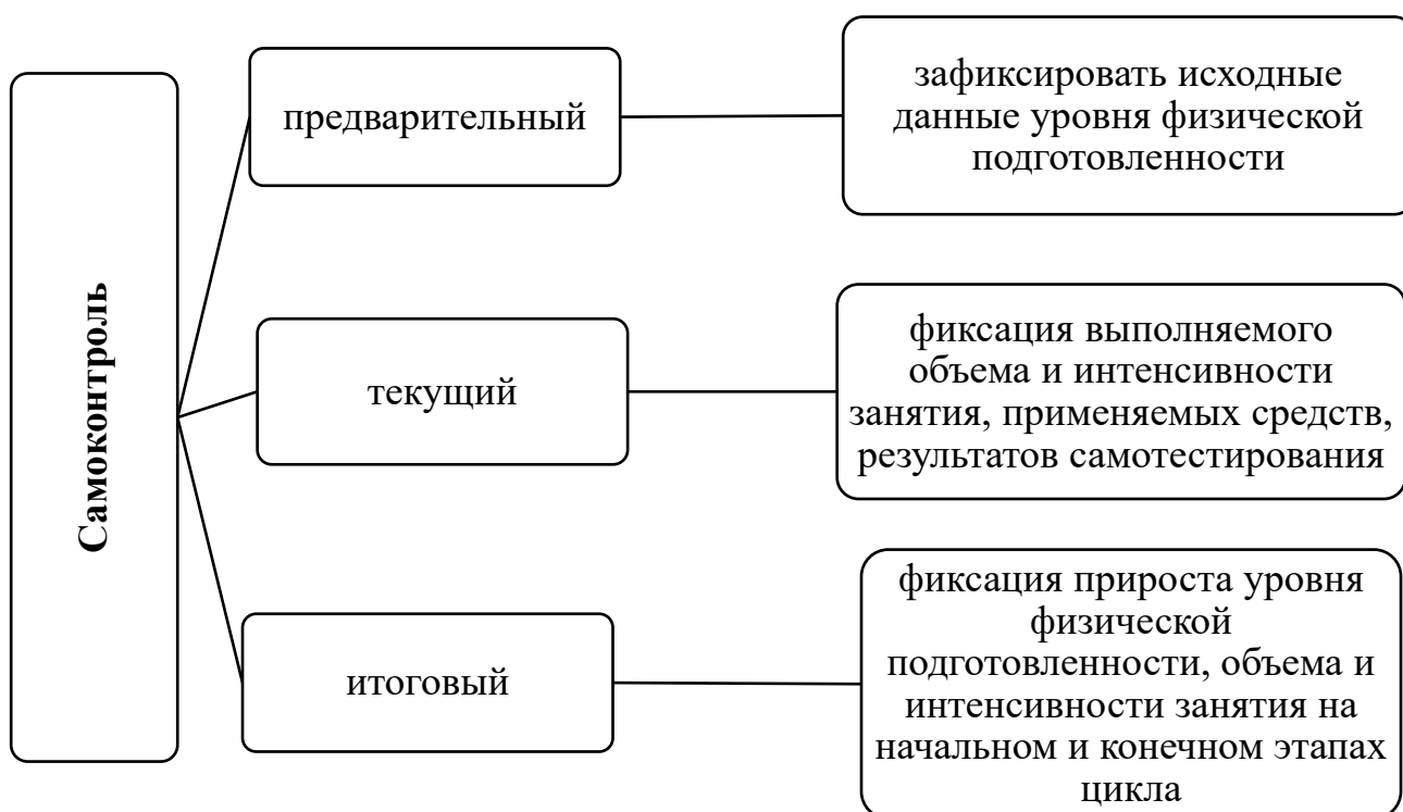
Рисунок 2 – Виды самоконтроля
